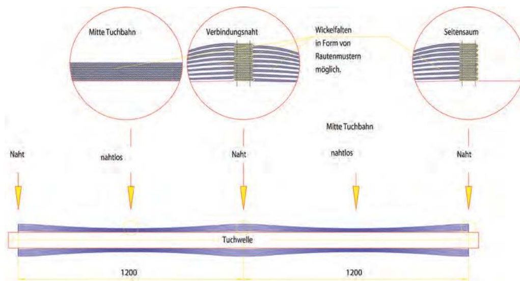
Bild 9.1.11 Unterschiedlicher Wickeldurchmesser im Naht- und Saumbereich
